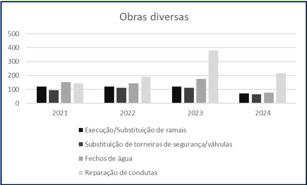
Gráfico - Intervenções na rede de abastecimento de água
